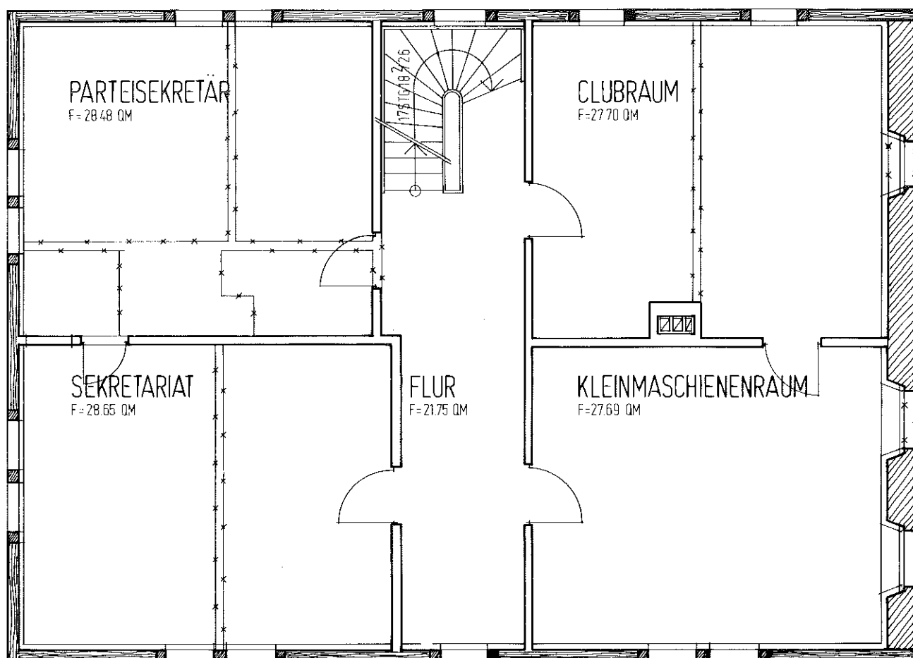
79 Grundriß 1. Obergeschoß
